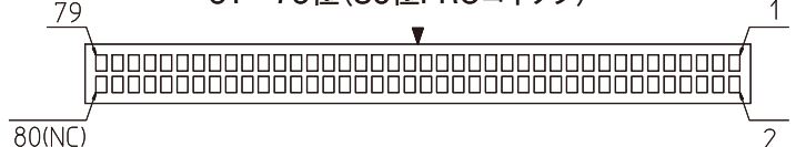
61~79極(80極FRCコネクタ)
