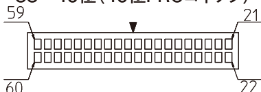
33~40極(40極FRCコネクタ)
